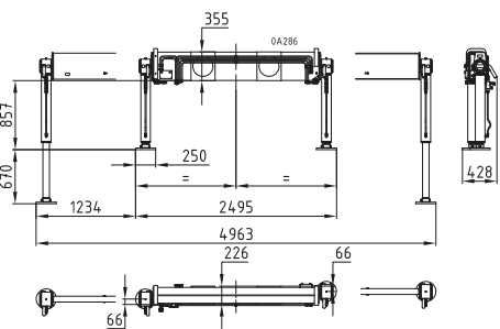
Schwenkabstützung breit / slewing outrigger wide
