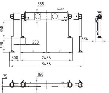
Schwenkabstützung / slewing outrigger
