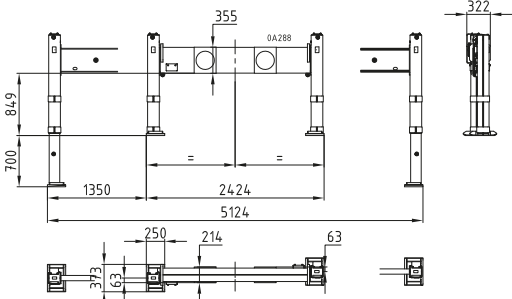
Vierkantabstützung breit / squared outrigger wide
