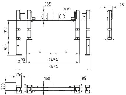
Vierkantabstützung / squared outrigger
