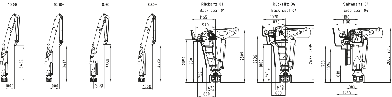
Schwenkabstützung / slewing outrigger
