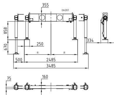
Schwenkabstützung / slewing outrigger
