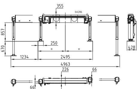
Schwenkabstützung breit / slewing outrigger wide
