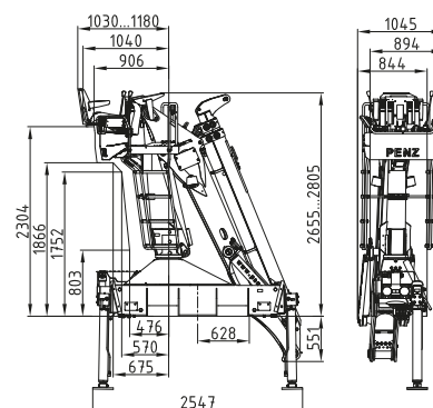
Rücksitz 04 mit Armsystem 10.40 Back seat 04 with load booms 10.40
