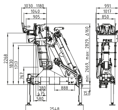
Rücksitz 04 mit Armsystem 8.70 Back seat 04 with load booms 8.70
