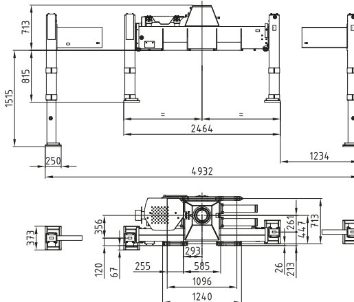
Vierkantabstützung Squared outrigger
