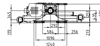
Seitensitz 04 Side seat 04
