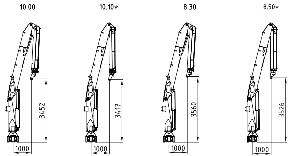
Vierkantabstützung / squared outrigger
