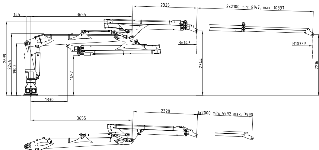
Kransockel stationär Crane base stationary
