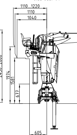
Seitensitz 04 Side seat 04
