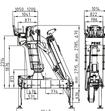
Rücksitz 04 mit Armsystem 9.50 Back seat 04 with load booms 9.50
