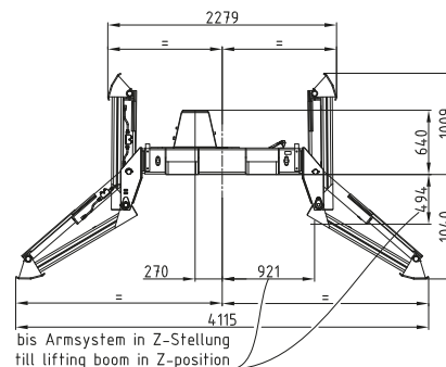
Klappabstützung Folding support
