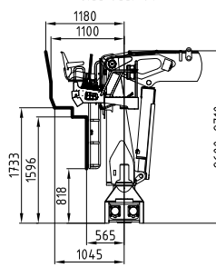
Seitensitz 04 Side seat 04
