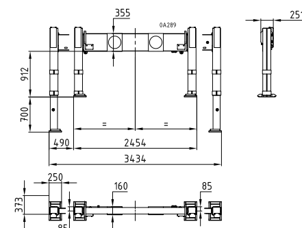
Vierkantabstützung breit / squared outrigger wide
